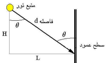
شکل (۸) روشنایی روی سطح عمود تحت زوایای مختلف
