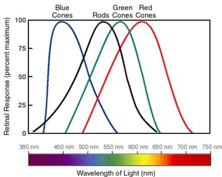
شکل (۱۳) مقایسه حداکثر حساسیت گیرنده‌های حسی سیستم بینایی
