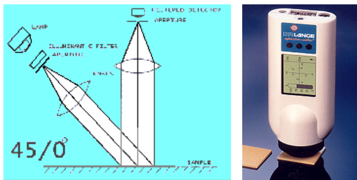
شکل (۱۲) نحوه تابش و نمونه دستگاه‌های رفلکتو اسپکترومتر
