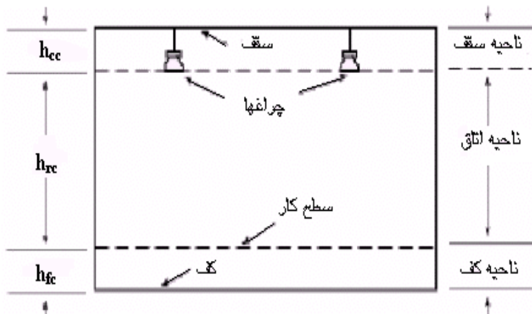
شکل (۲۲) مبنای تعیین ارتفاع طراحی و ارتفاع ناحیه فضای سقف و ناحیه کف
