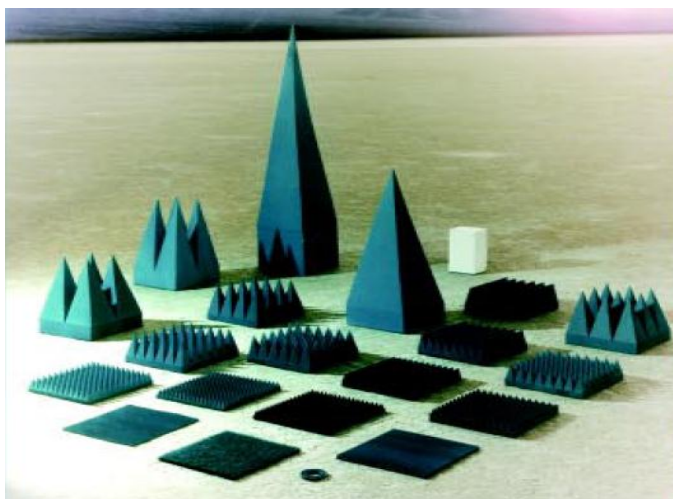
شکل ۵۶- جاذب‌های دی‌الکتریک امواج با شکل ظاهری هرمی
