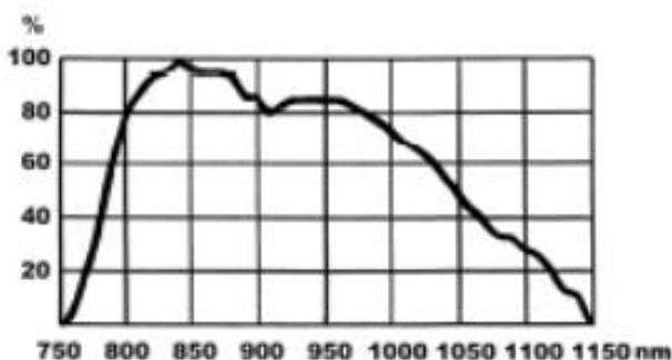
شکل ۲۴ - نمونه رادیومتر اندازه‌گیری پرتو مادون قرمز نزدیک
