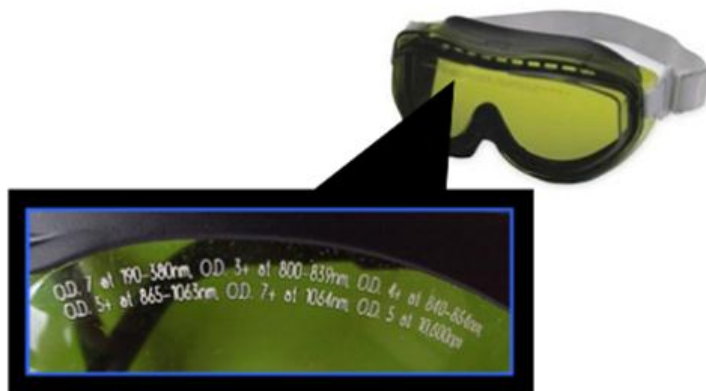
شکل ۷۲- عینک مخصوص محافظ لیزر با شناسنامه کاهندگی بر روی لنز
