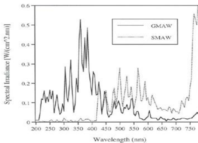
شکل ۱۵- تجزیه طیفی انواع جوشکاری برق با استفاده از اسپکترو رادیومتر
