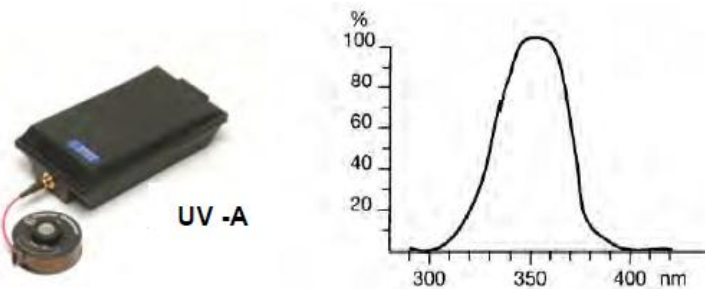
شکل ۱۳- منحنی حساسیت رادیومتر فرابنفش در محدوده UVA
