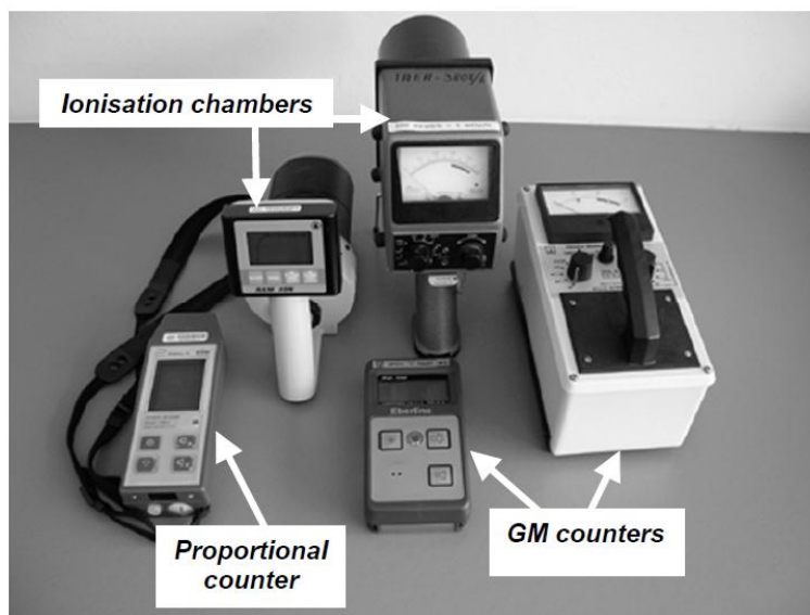
شکل ۷۹- انواع آشکارسازهای گازی جهت ارزیابی‌های محیطی پرتوهای یونیزان
