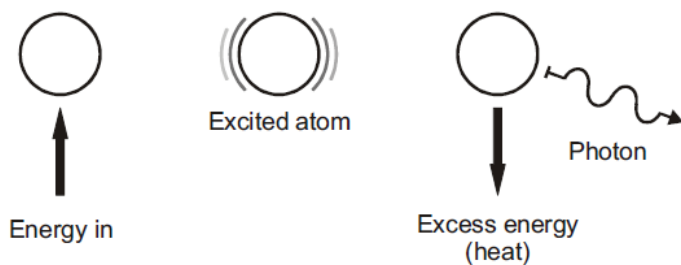
شکل ۵۸- برانگیختگی معمولی اتم‌ها و انتشار خودبه‌خودی فوتون
