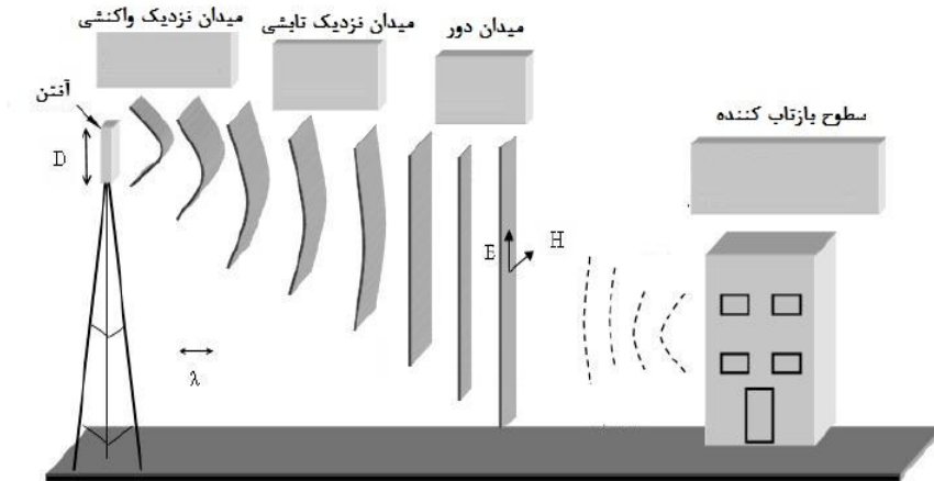
شکل ۲۷- نحوه انتشار امواج میکروویو از یک نمونه آنتن ارتباطی
