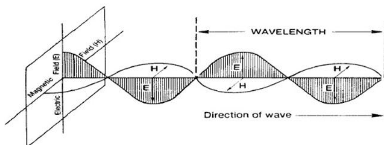
شکل ۲۶- انتشار موج الکترومغناطیس و برهم‌کنش میدان‌های الکتریکی (E) و مغناطیسی (H)
