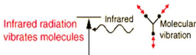
شکل ۲۱- مکانیسم اصلی اثرگذاری پرتو مادون قرمز
