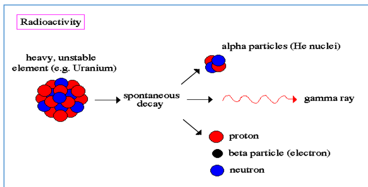
شکل ۷۵- واپاشی هسته مواد رادیواکتیو منشأ ایجاد پرتوهای یونیزان
